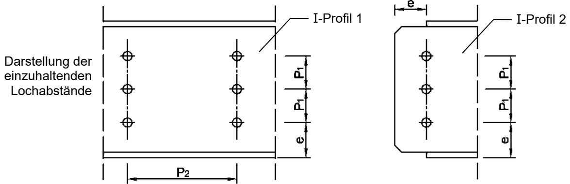
Ansicht B (ohne Darstellung des L-Profils)
