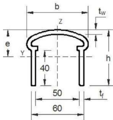
Handlauf 64 x 70
