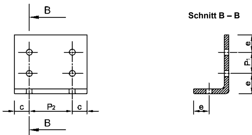
L-Verbindungs-Profil mit Darstellung der einzuhaltenden Lochabstände
